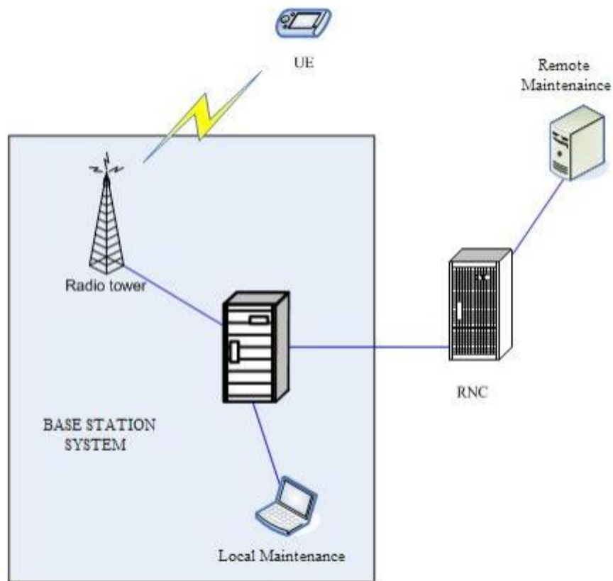
Сурет 3.6 - ZTE базалық станциясының құрылымы
