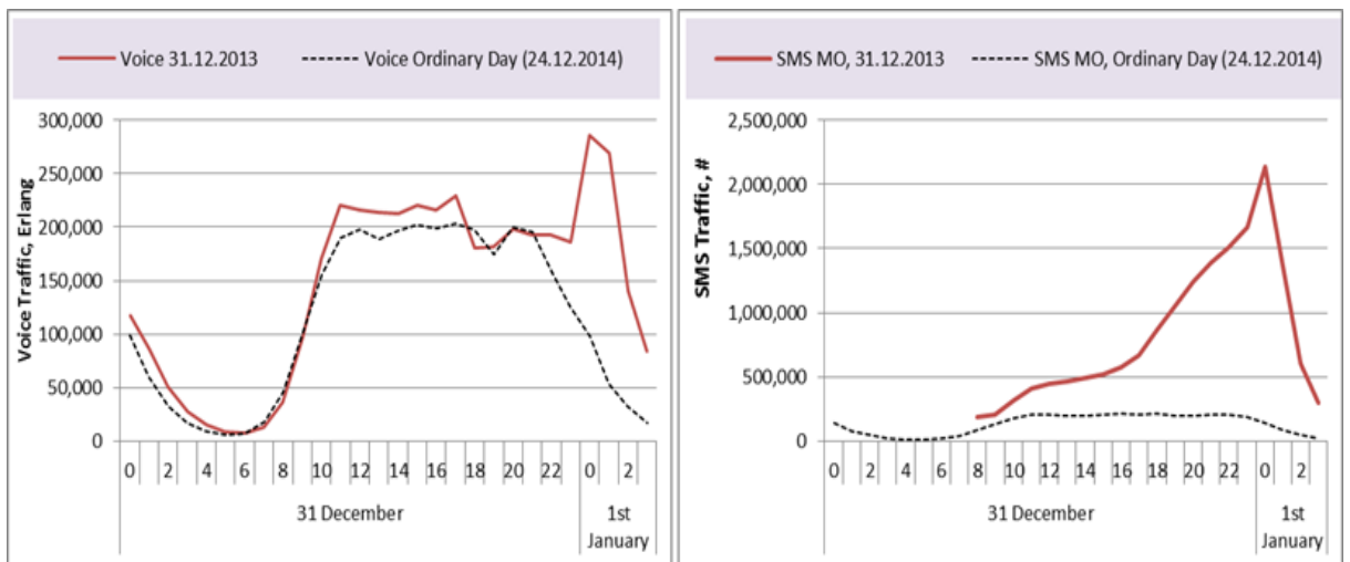
Сурет 3.11 – (Voicetraffic/SMSTraffic) ұялы байланыс желісінің өнімділігінің статистикалық деректері
